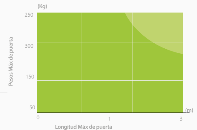
Diagrama límite de utilización
