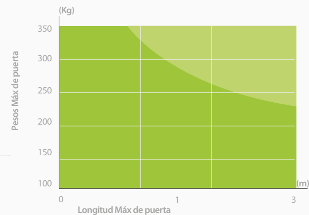
Diagrama límite de utilización
